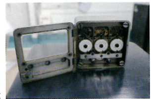
現代の時間錠の内部構造
